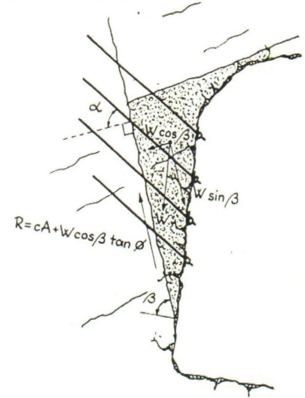
H.5. Gia cố khối nêm trượt
