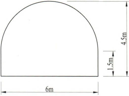
H.6. Kích thước mặt cắt ngang đường hầm
