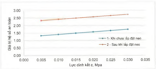
H.11. Biểu đồ quan hệ giữa lực dính kết c (MPa) và Giá trị hệ số an toàn của khối nêi phía nóc số 8
