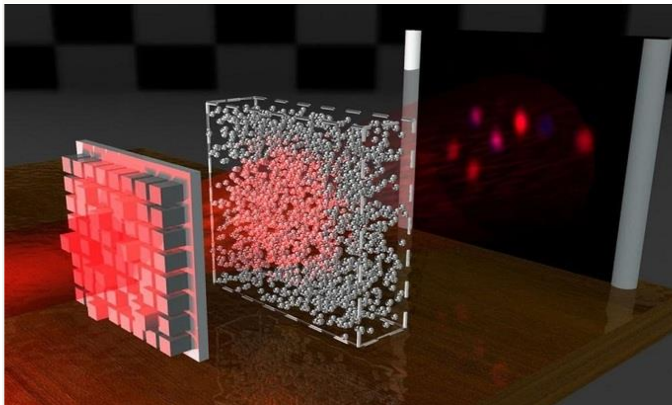
Mô phỏng ánh sáng truyền qua các hạt nano của lớp bột oxit kẽm.
